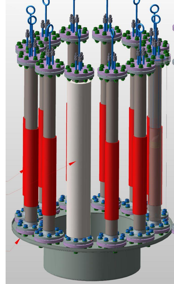
Kaavakuva koelaitteistosta: yhteensä 12 kpl 4,2 l paineastiointia, 3 kpl käytössä tässä kokeessa
